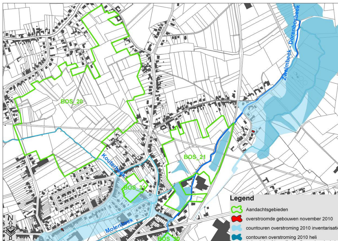
Figuur 10: Situering op OWKM/modelleringsstudie
