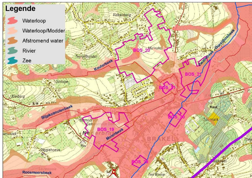
Figuur 8: Situering op NOG-kaart
