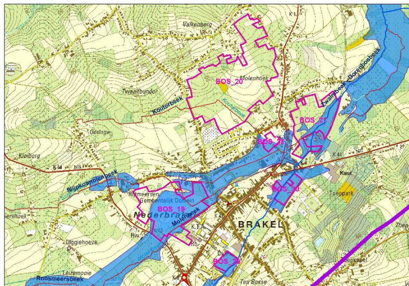
Figuur 9: Situering op ROG-kaart
