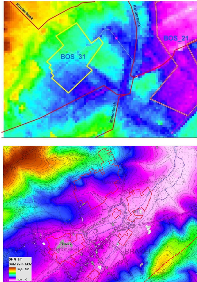
Figuur 11 a + b: Situering op DHM
