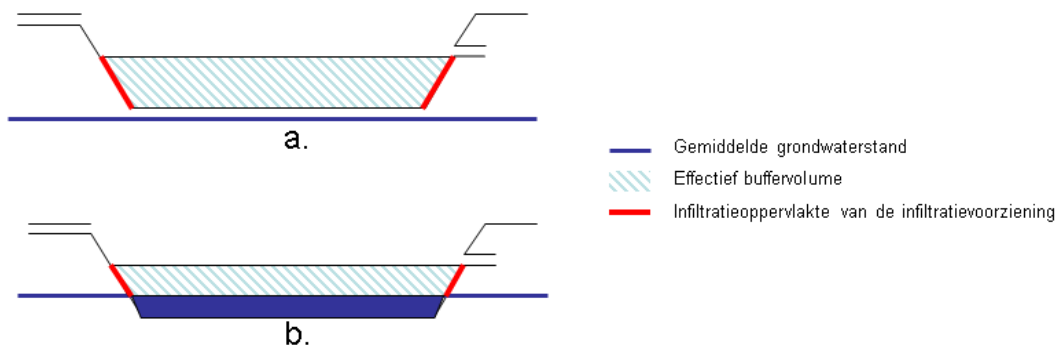
Figuur a: Aanleg van een infiltratiebekken boven de grondwaterafel Figuur b: Aanleg van een infiltratiebekken dat zich gedeeltelijk onder de grondwaterafel bevindt, waardoor het effectief buffervolume kleiner is
