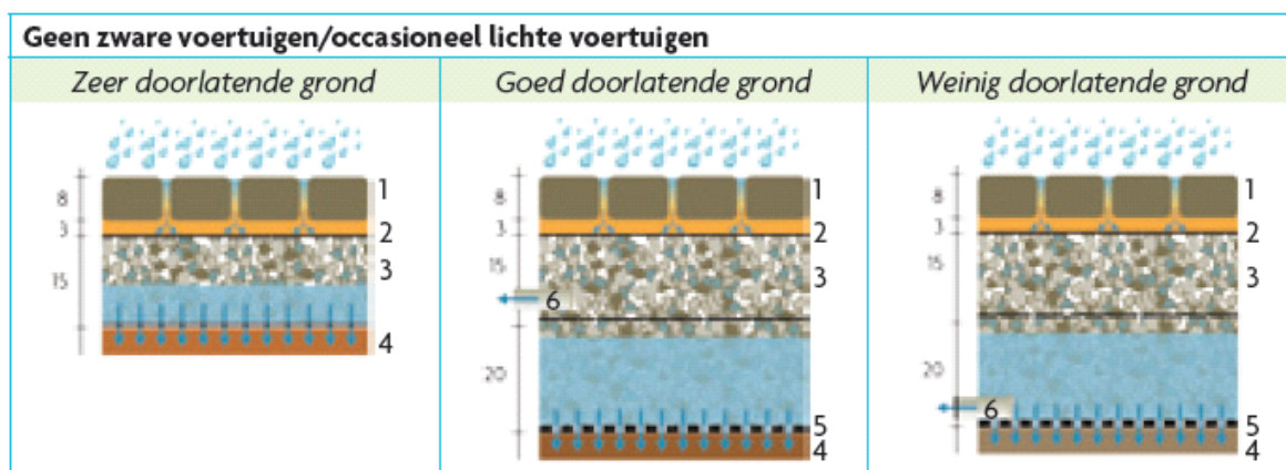
Figuur 3.3 : opbouw van een waterdoorlatende verharding
